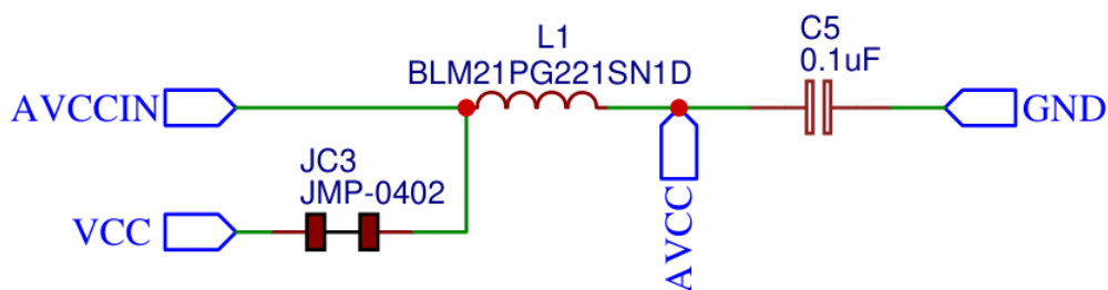
Рисунок 12 – Схема подачи питания аналоговых блоков
